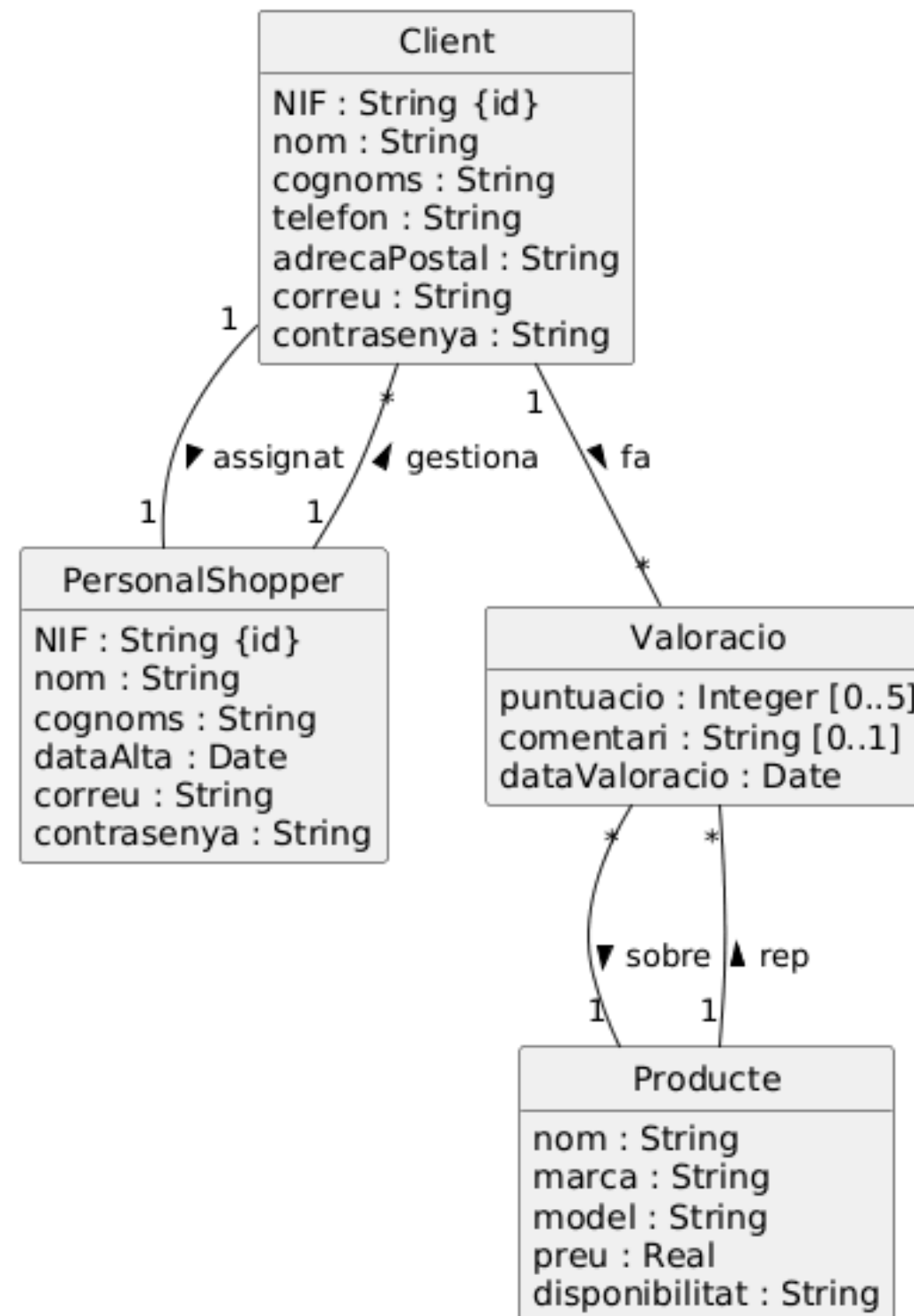
Diagrama de Classes: Sistema de valoracions
