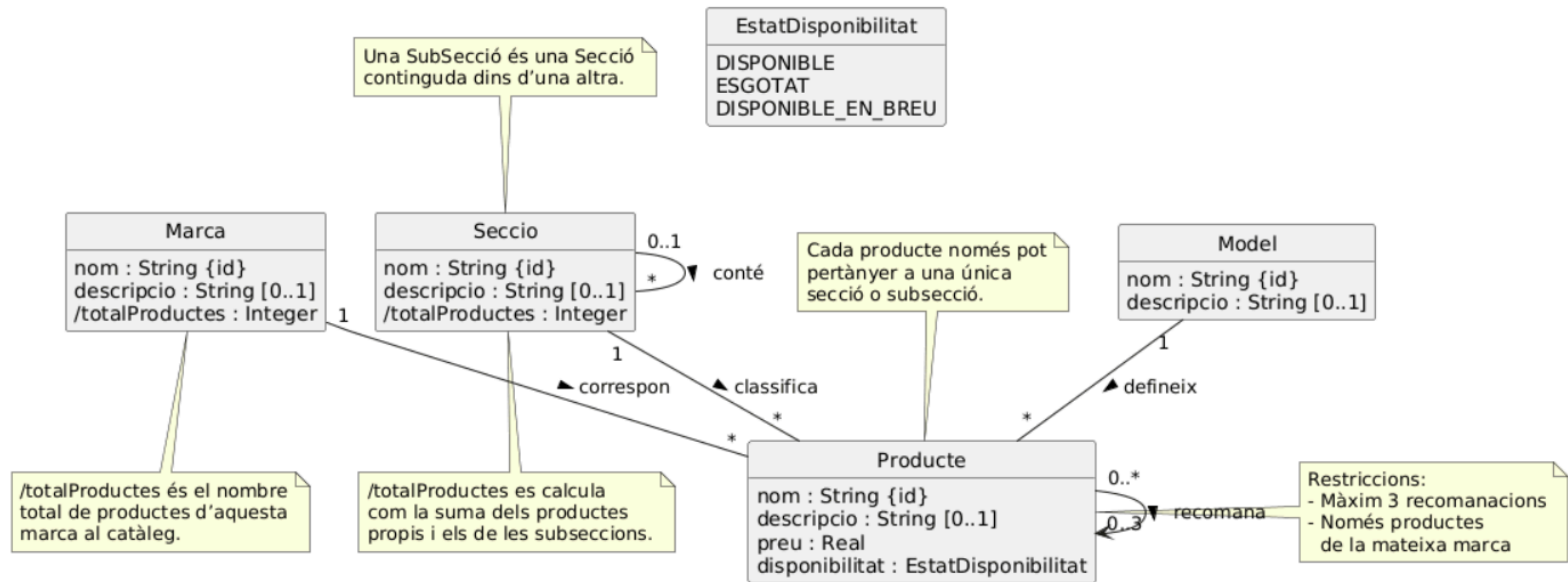
Diagrama de Classes: Model de Domini del Catàleg de Productes
