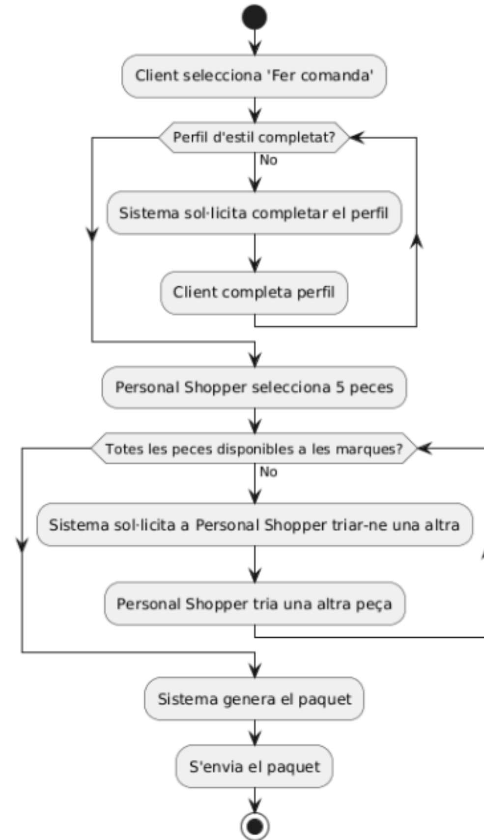
Diagrama d'Activitat: CU02 Fer una comanda
